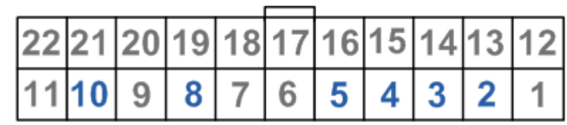
WIDOK OD PRZODU URZĄDZENIA
